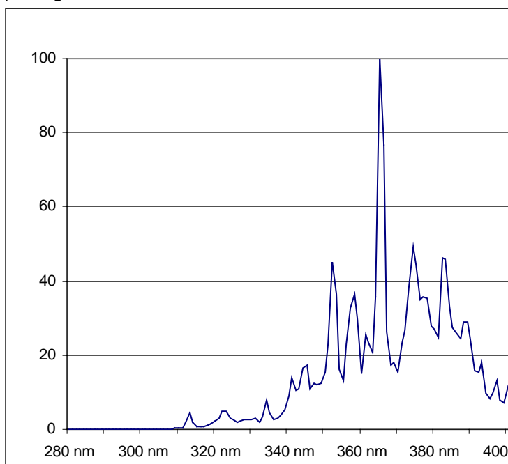
Rel. spektraler Strahlenfluss / Rel. Spectral Radiant Flux
